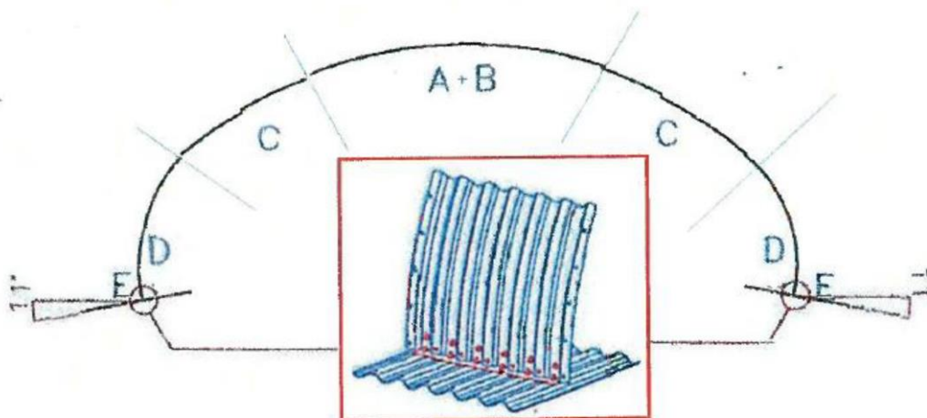
Rys. 1 Przygotowanie spągu pod ułożenie fundamentów ze stalowych blach falistych.
